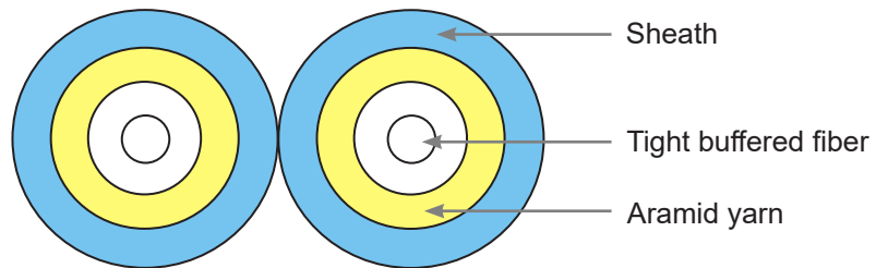
OM3 Cable
