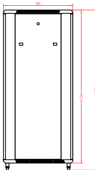
SIDE DOOR
